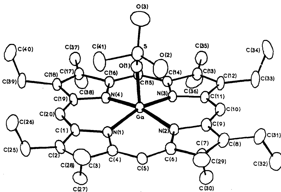
Fig. 2. Vue ORTEP du complexe [Ga(OEP)(SO_3CH_3)] ( III_{1a} ).
