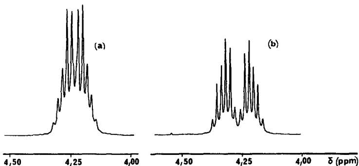
Fig. 1. Signaux de résonance des protons méthyléniques du complexe [\text{Ga}(\text{OEP})(\text{SO}_3\text{CH}_3)] ( \text{III}_{1\text{a}} ): (a) dans \text{CDCl}_3 ; (b) dans \text{C}_6\text{D}_6 .
